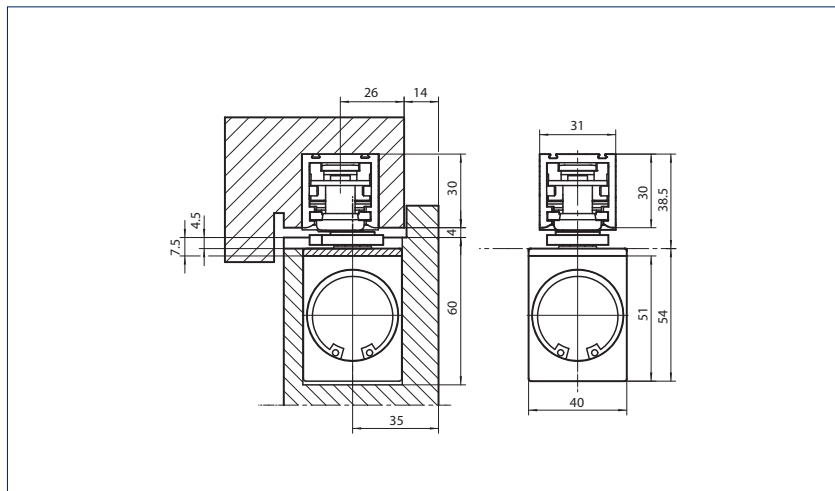
Fig. 10-2 · Размеры - GEZE Boxer, сила закрывания 3-6 (ISM/E-ISM на деревянной двери с упором дверной створки)
