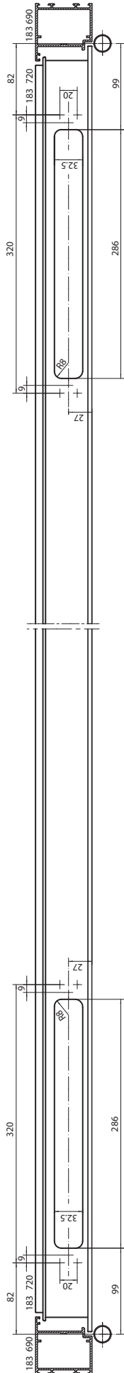
Fig. 14-1 · Скользящая шина ISM/E-ISM Boxer - сила закрывания 2-4/3-6, алюминиевая дверь Интернет магазин дверных доводчиков DOORK-SHOP.RU Заказ и консультации: Телеф: +7 (499) 502-80-00
