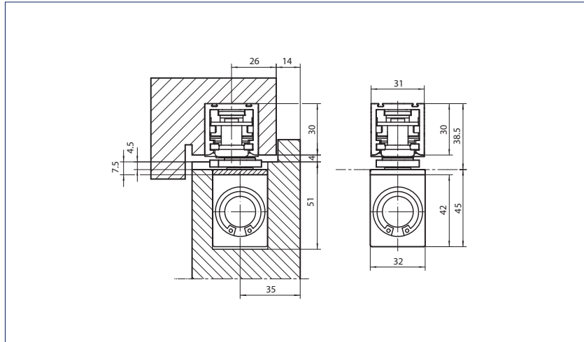
Fig. 10-1 · Размеры - GEZE Boxer, сила закрывания 2-4 (ISM/E-ISM на деревянной двери с упором дверной створки)
