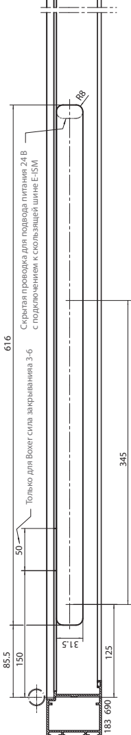
Fig. 14-1 · Скользящая шина ISM/E-ISM Boxer - сила закрывания 2-4/3-6, алюминиевая дверь Интернет магазин дверных доводчиков DOORK-SHOP.RU Заказ и консультации: Телеф: +7 (499) 502-80-00
